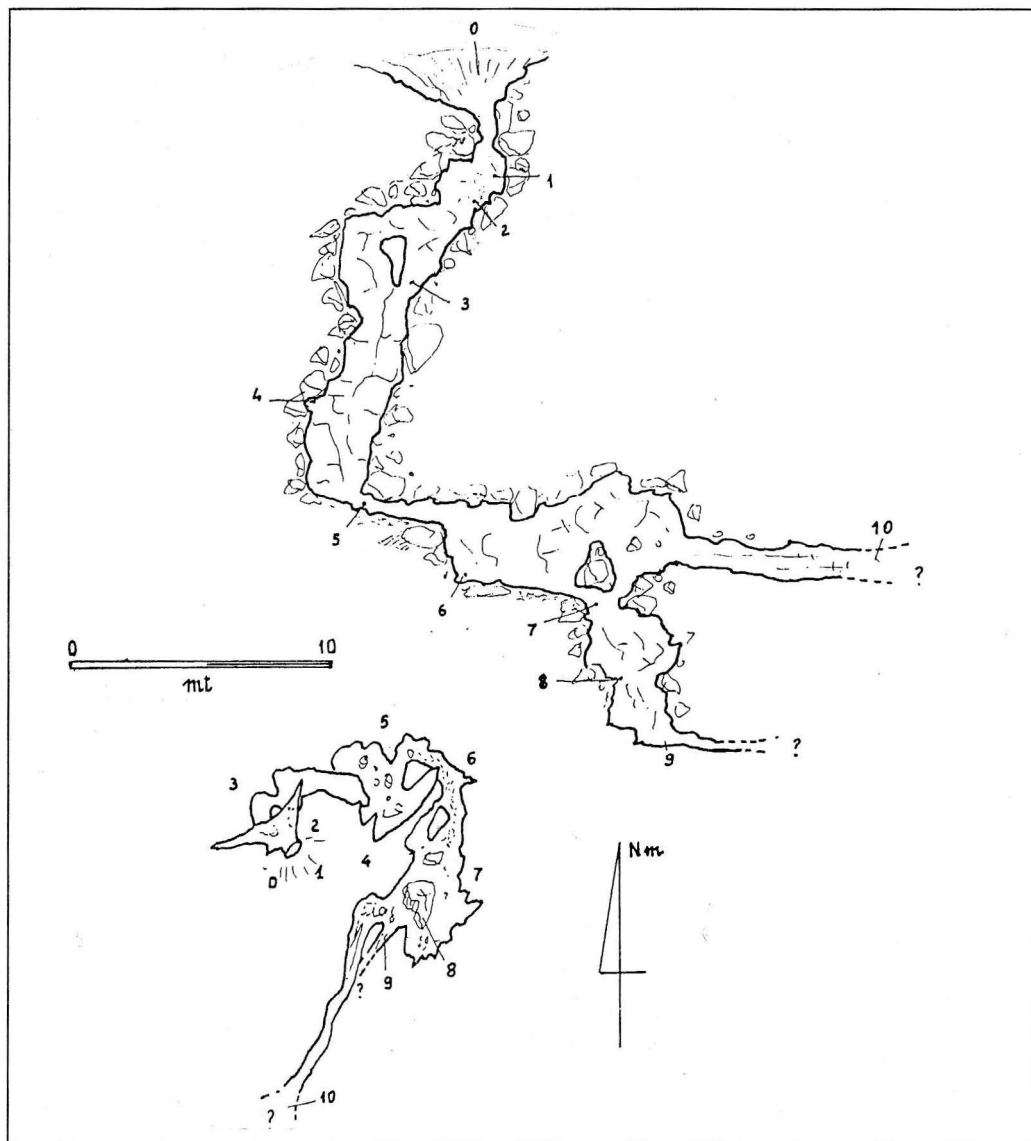
Inghiottoitoio 3° as Ovest del Figliolo. Rilievo 10-8-88 - P. Giuliani, C. Fusilli - Gruppo Speleologico Dau- no - F.G. A.I.R.E.S.
